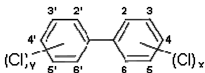
Figura 3 Struttura generale dei PCB
