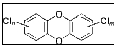
Figura 1 Struttura generale delle PCDD
